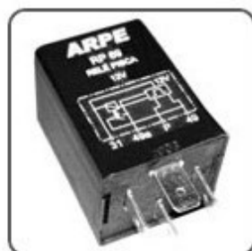
RP69 - FIAT RELÉ DE PISCA 12V - 400W 4 TERMINAIS LÂMPADA PILOTO
