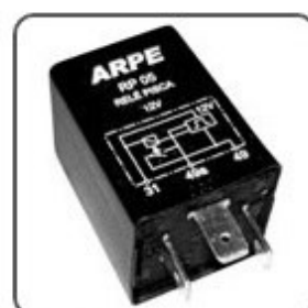
RP05A - UNIVERSAL, VÁRIOS CLIENTES RELÉ DE PISCA 12V - 400W - FIXAÇÃO POR ADESIVO
