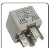
RA9022 - GM RELE DE COMANDO DO AR CONDICIONADO DUPLA NA - 12V 20/12A, 6 TERMINAIS - ORIGINAL
